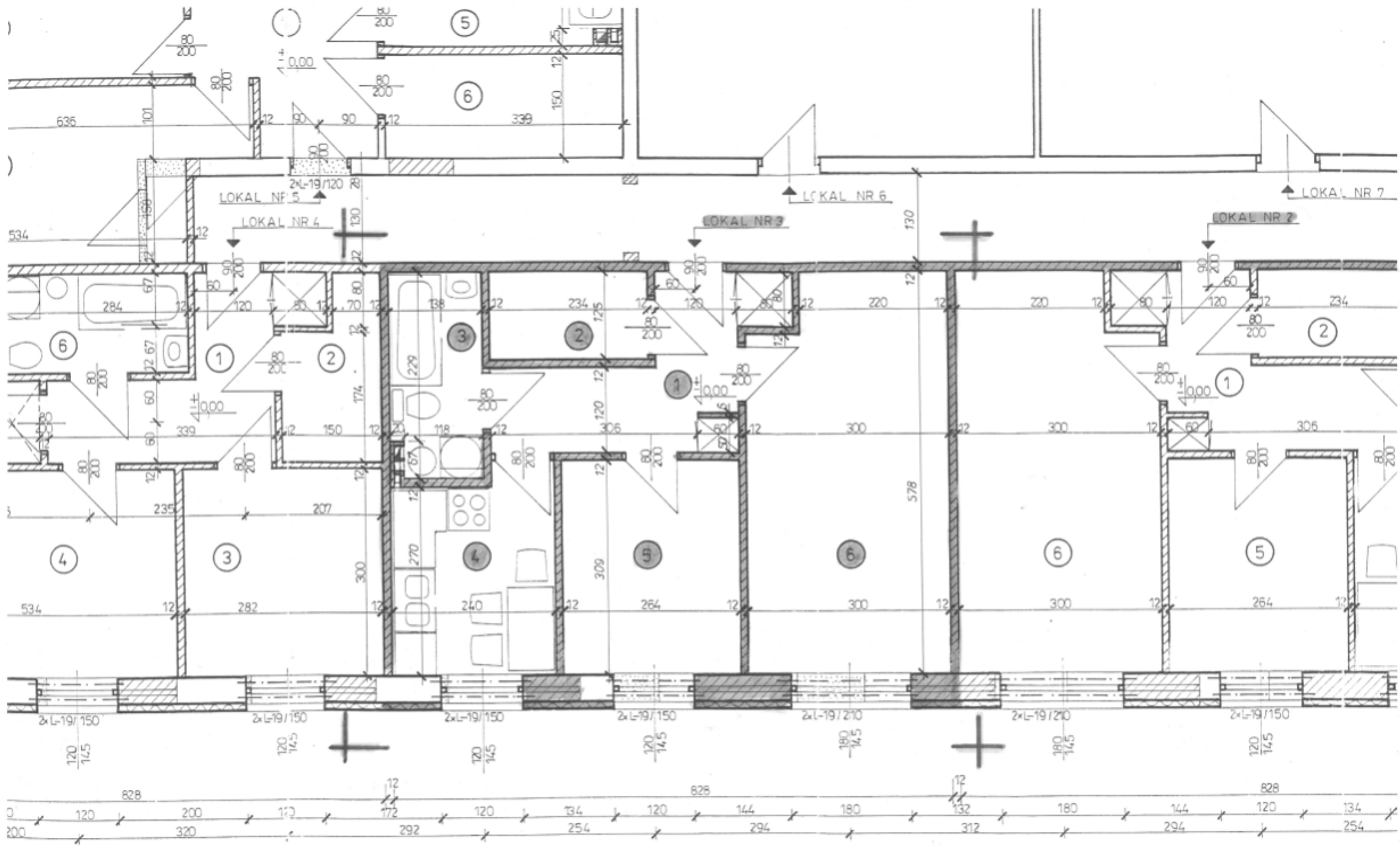
Rzut parteru - fragment
